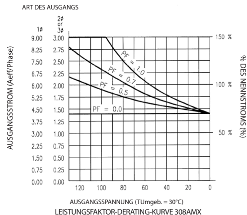
AUSGANGSSPANNUNG – WECHSELSPANNUNGSEFFEKTIVWERT Kurzzeitige Überlastungen bis 150% sind zulässig. Die Betriebsdauer bis zur thermischen Abschaltung oder bis zum Auslösen der Schutzschalter kann abhängig von den Leitungs- und Temperaturbedingungen von wenigen Sekunden bis zu einigen Minuten dauern.
